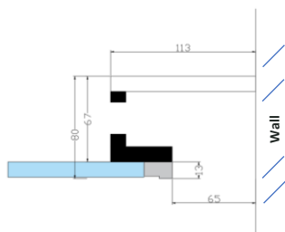
Return grille
